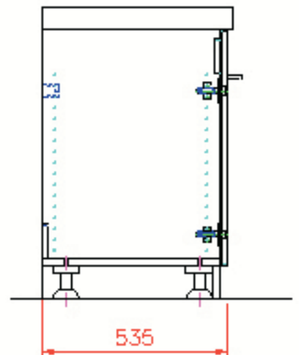
Schul-Waschtisch Mod. Nr. 162700 mit Unterschrank aus KF weiss Tür mit Bügelgriff (rechts angeschlagen)
